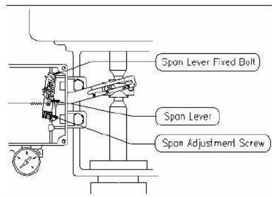
Ação Direta
